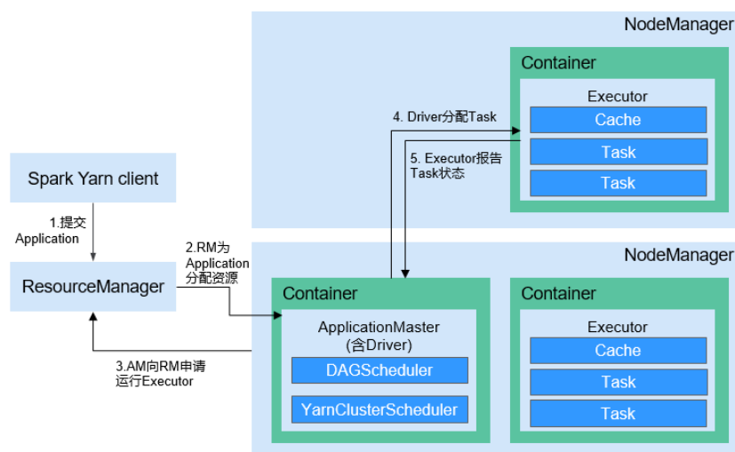
图 1-131 Spark on yarn-cluster 运行框架
