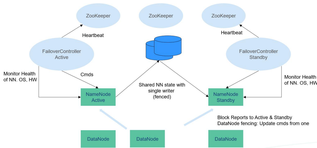
图 1-46 典型的 HA 部署方式
