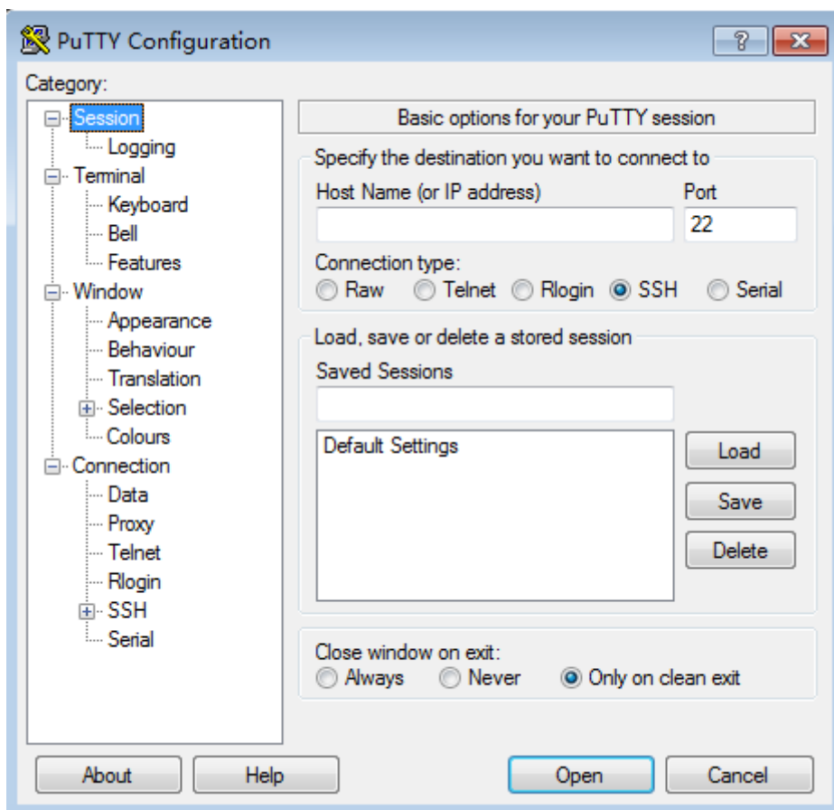
图 9-2 单击 Session
