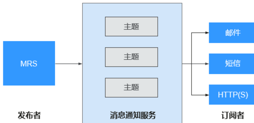
图 1-144 实现过程
