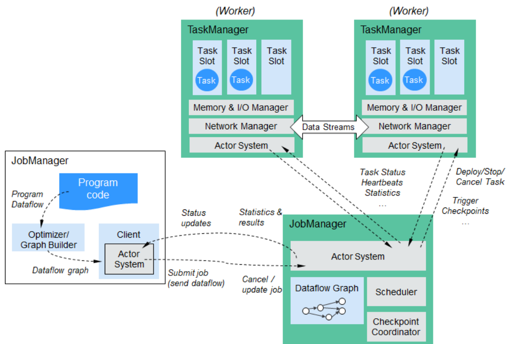
图 1-12 Flink 结构
