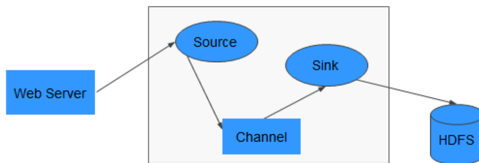
图 1-28 Flume-NG 架构
