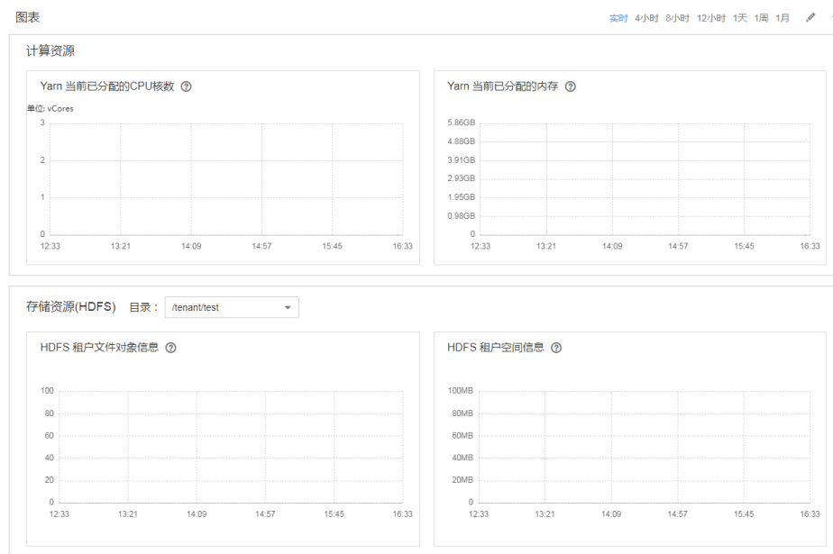
图 12-15 精细化监控
