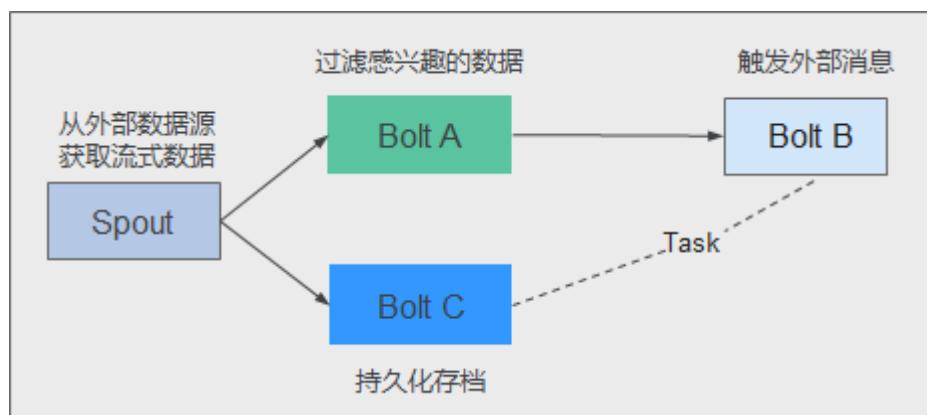
图 1-124 Topology
