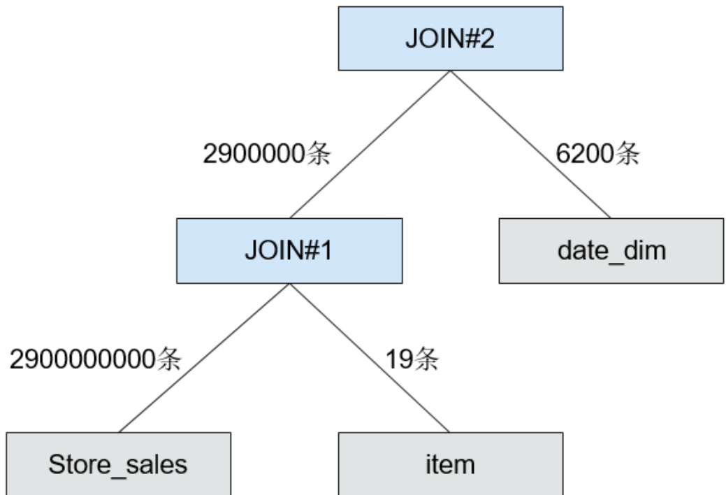
图 1-63 开启 CBO
