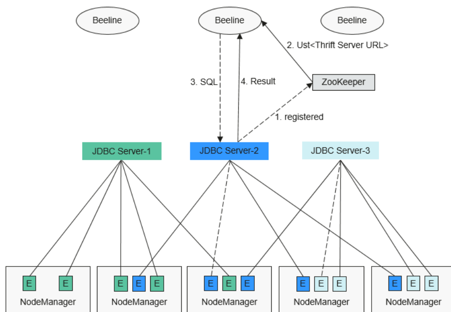
图 1-97 Spark JDBCServer HA
