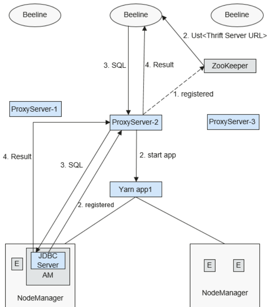
图 1-116 Spark JDBCServer 多租户
