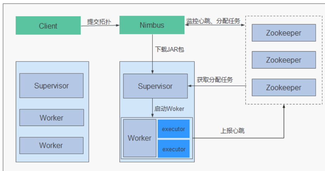
图 1-123 Storm 系统架构
