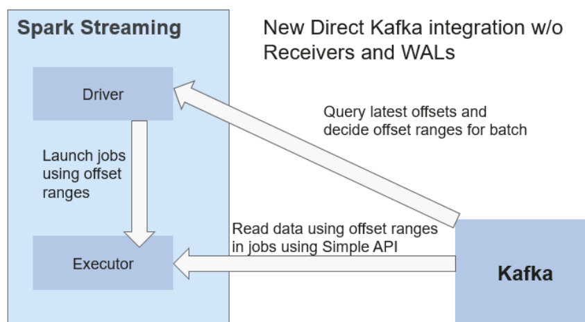
图 1-88 Direct Kafka 接口数据传输
