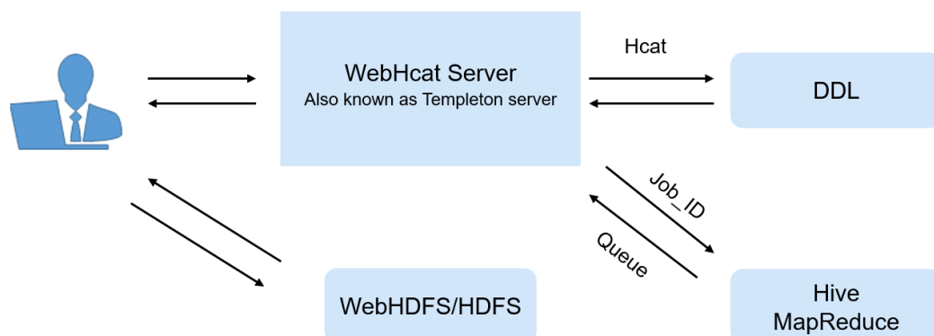
图 1-58 WebHCat 的逻辑架构图
