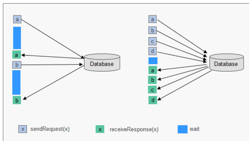
图 1-27 Async.I/O 的比较
