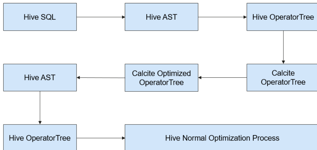
图 1-60 实现流程图
