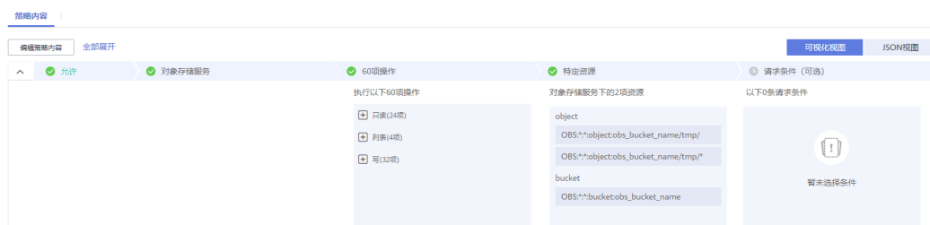
图 18-57 自定义策略
