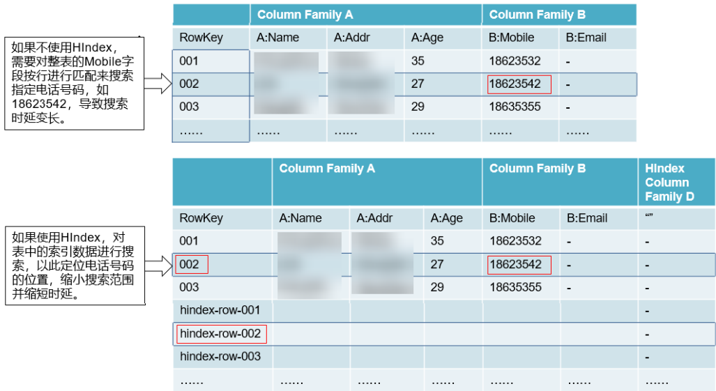
图 1-39 HIndex
