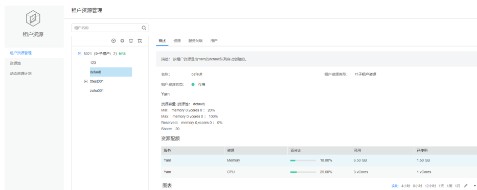
图 12-14 多租户管理
