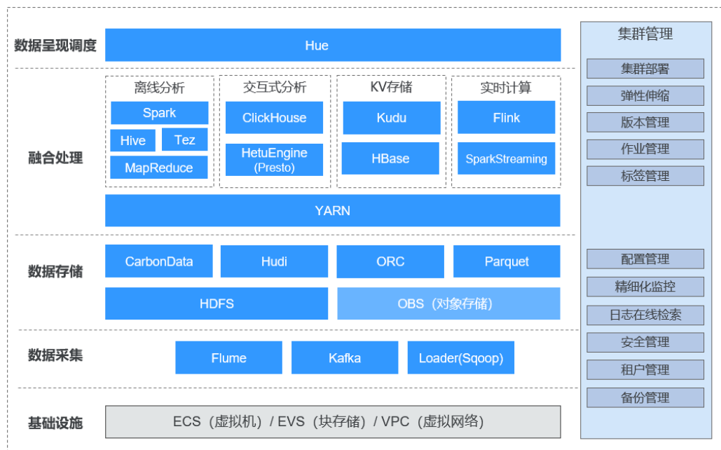
图 1-1 MRS 架构
