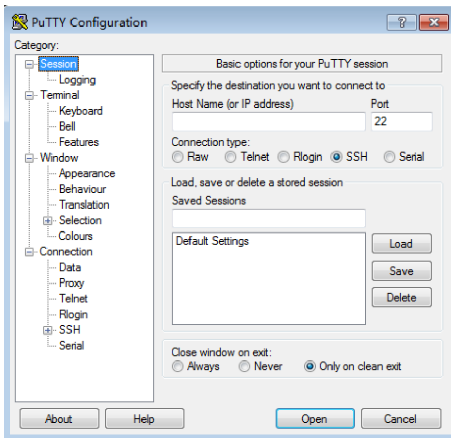
图 9-1 单击“Session”
