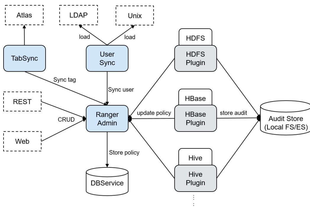
图 1-83 Ranger 结构
