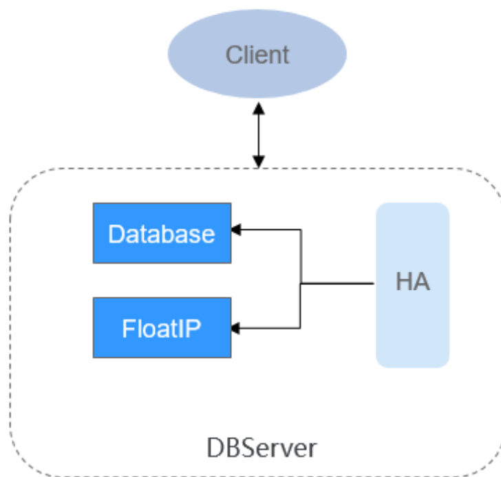
图 1-10 DBService 结构
