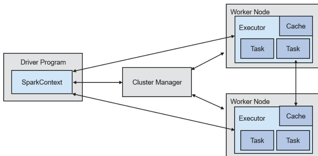
图 1-85 Spark 结构
