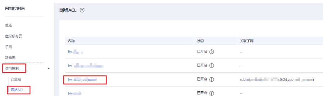
图 5-1 网络 ACL
