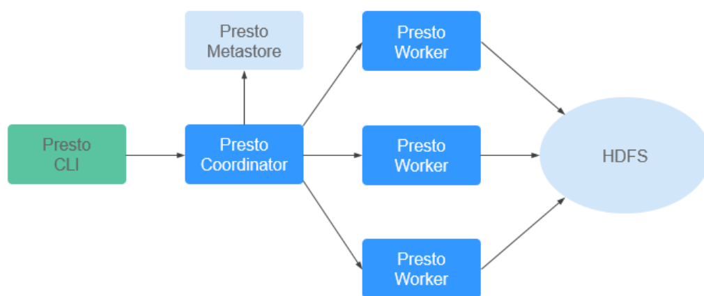
图 1-82 Presto 架构
