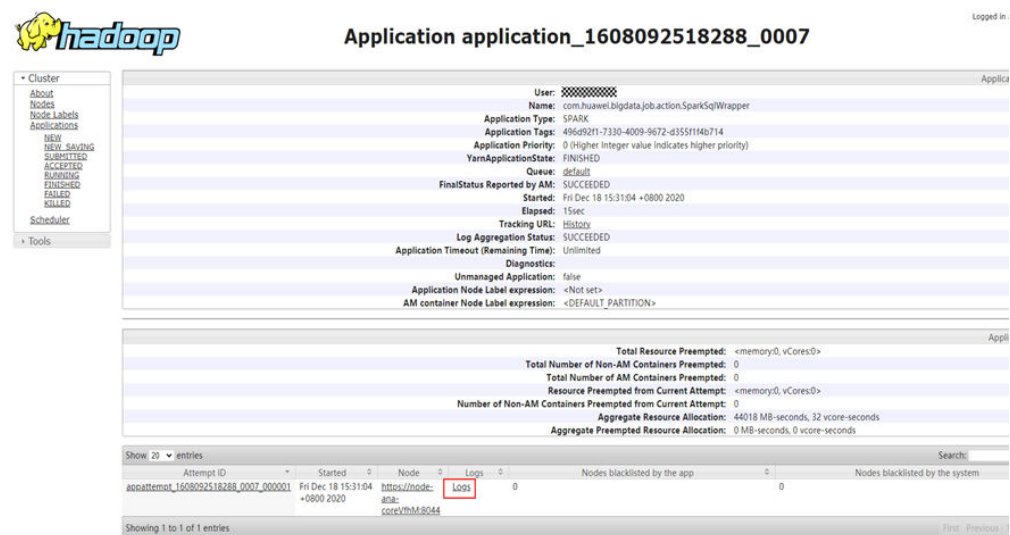
图 18-8 任务日志
